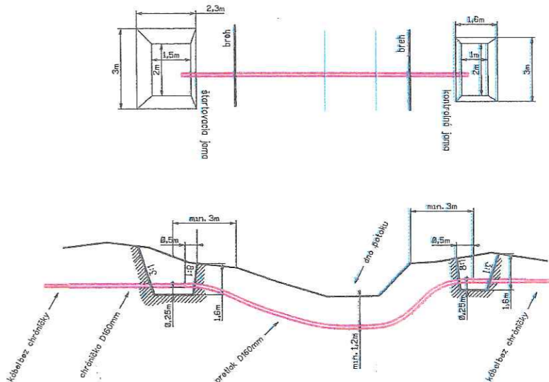
Riadený pretlak pod Gánovským potokom (ID 4-32-01-3310): M 1:250
